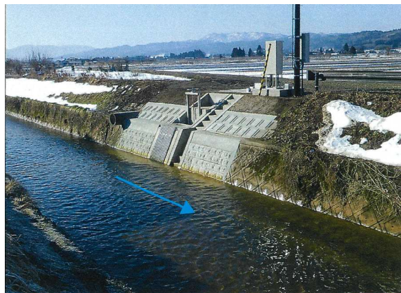
揚水機全景(栗村用水路)
